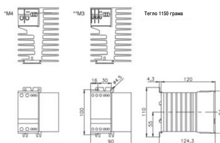
Размери за модул 90 мм (LAS2 50 A/63 A/LAA 50 A)
