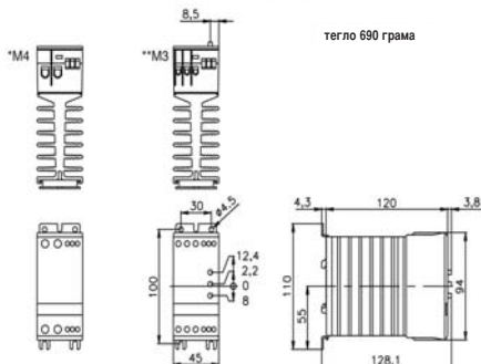
Размери за модул 45 мм (LAN)
