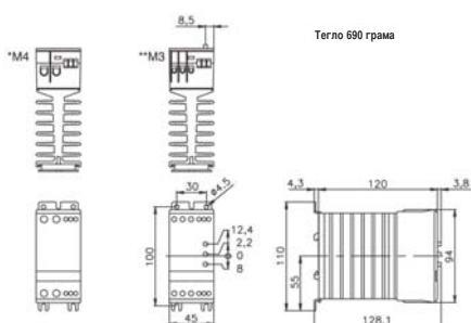
Размери за модул 45 мм (LAS1/LAW/LAK15A/LAD/LAA 30 A)
