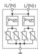
Вътрешна схема BV25
