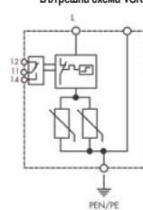
Вътрешна схема VSR
