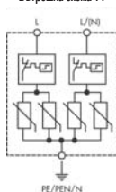
Вътрешна схема VV
