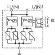
Вътрешна схема BV25R
